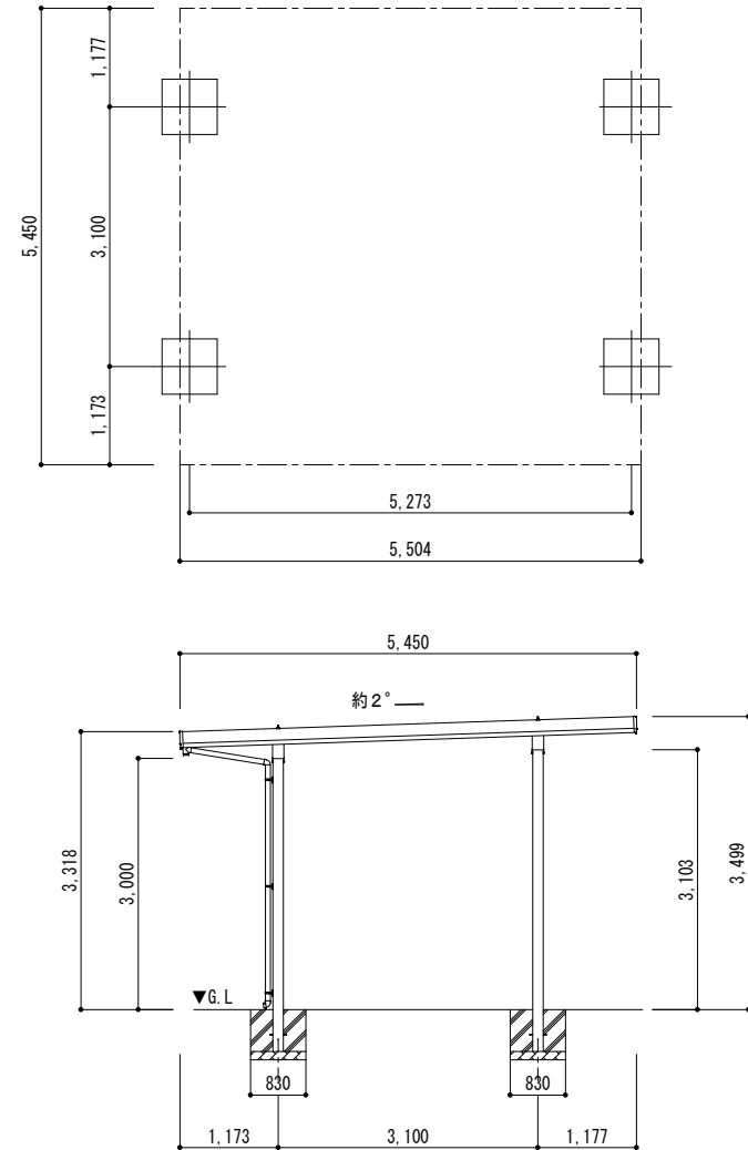
■基礎配置図
